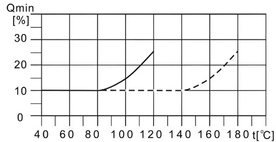
Рисунок – 7. График зависимости минимального расхода от температуры жидкости
