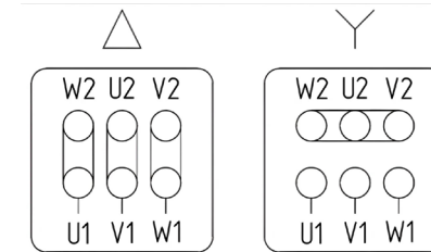
Рисунок – 11. Схема соединения обмоток электродвигателя
