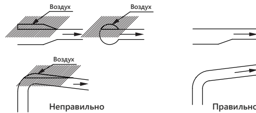
Рисунок – 10. Правильный монтаж трубопроводов
