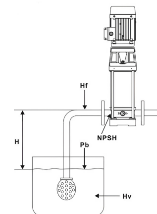
Рисунок – 6. Система с насосом
