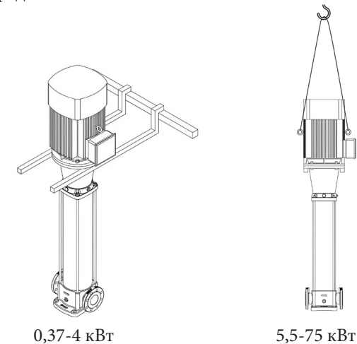
Рисунок – 9. Схема подъема насоса
