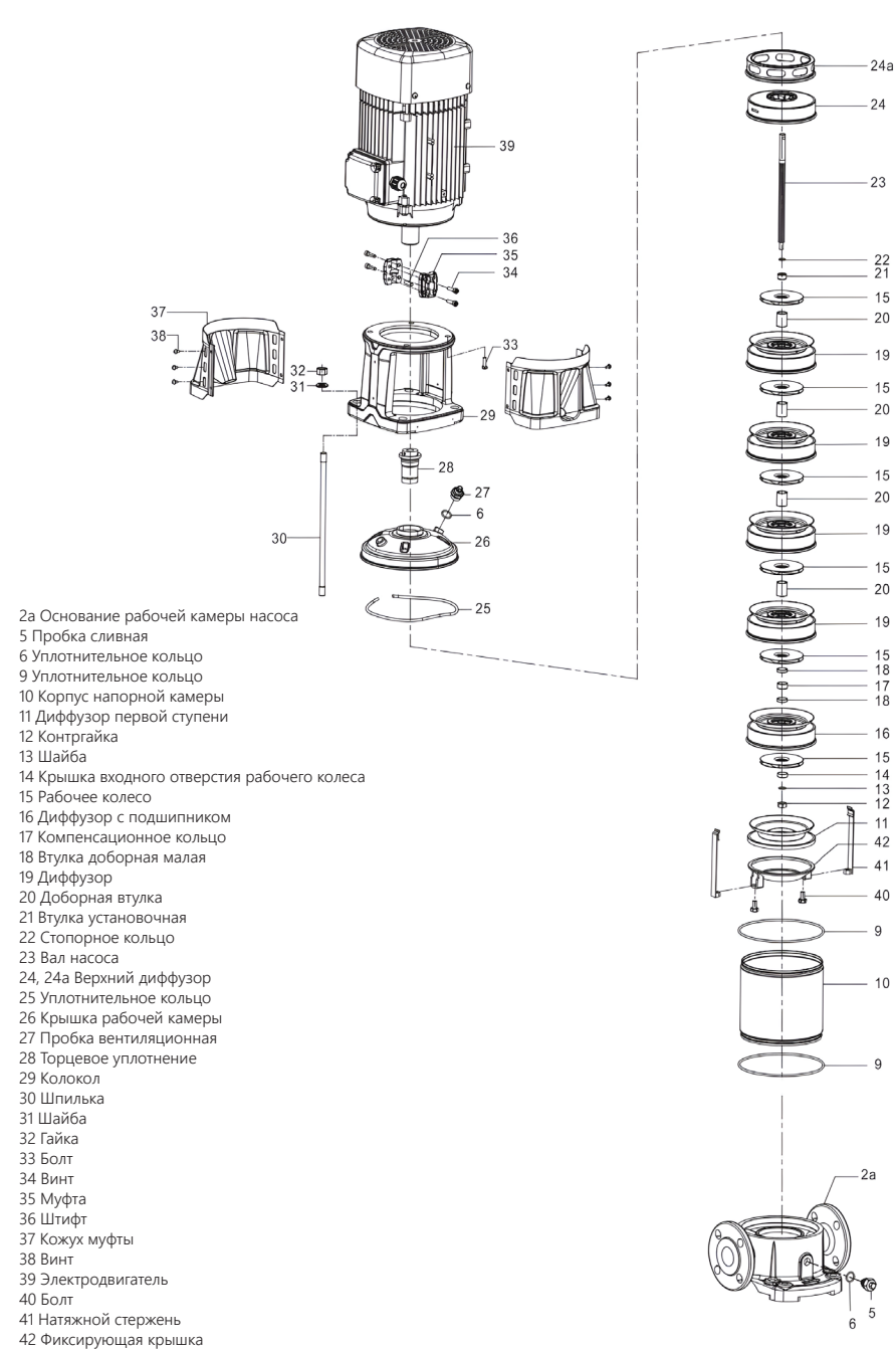
Рисунок – 4. Устройство насоса (BVP 10/15/16/20)
