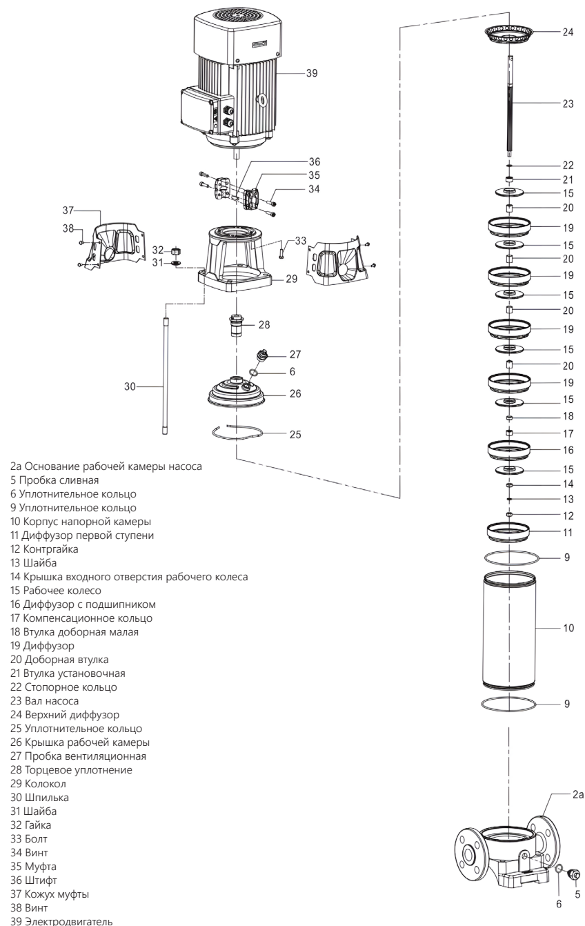
Рисунок – 3. Устройство насоса (BVP 1/2/3/4/5)
