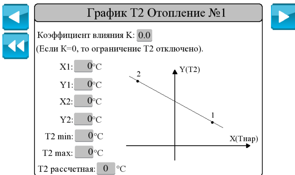
Рисунок 8 – Дисплей «График T2».
