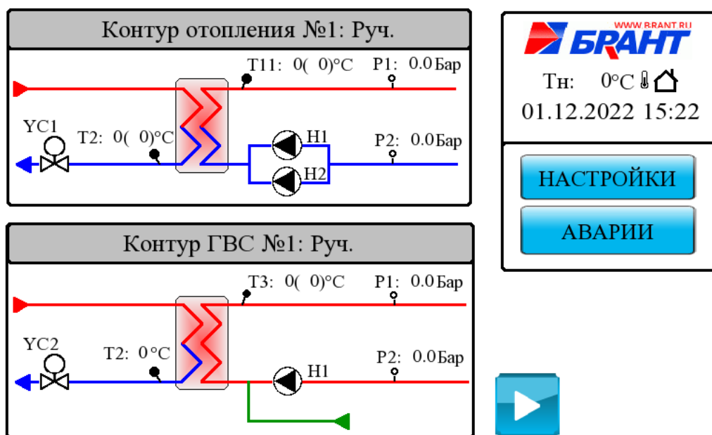
Рисунок 4 – Дисплей «Главное меню»
