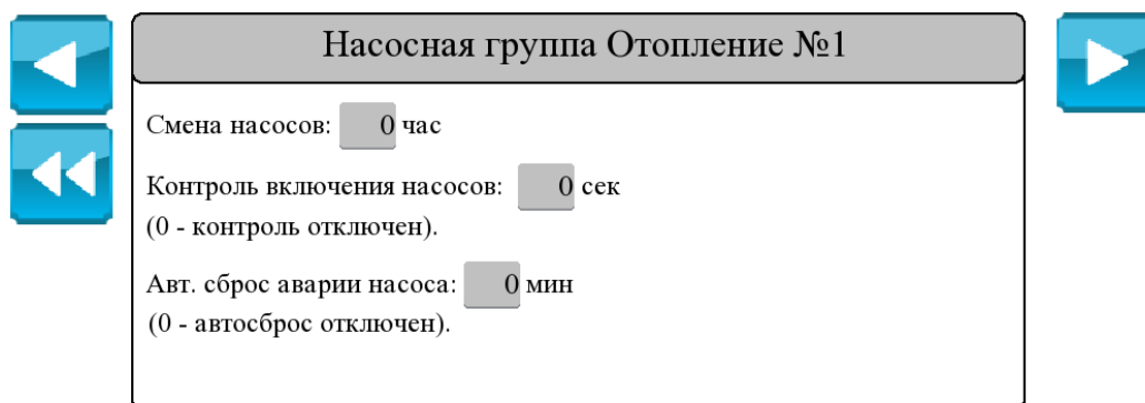
Рисунок 9 – Дисплей «Насосы»
