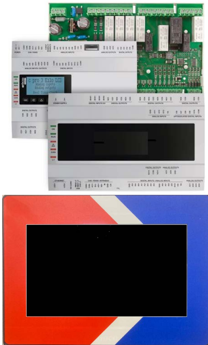
Рисунок 3 – Внешний вид плк и панели оператора.
