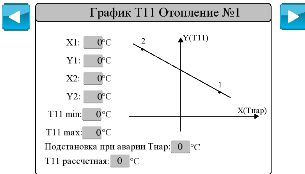
Рисунок 7 – Дисплей «График T11»
