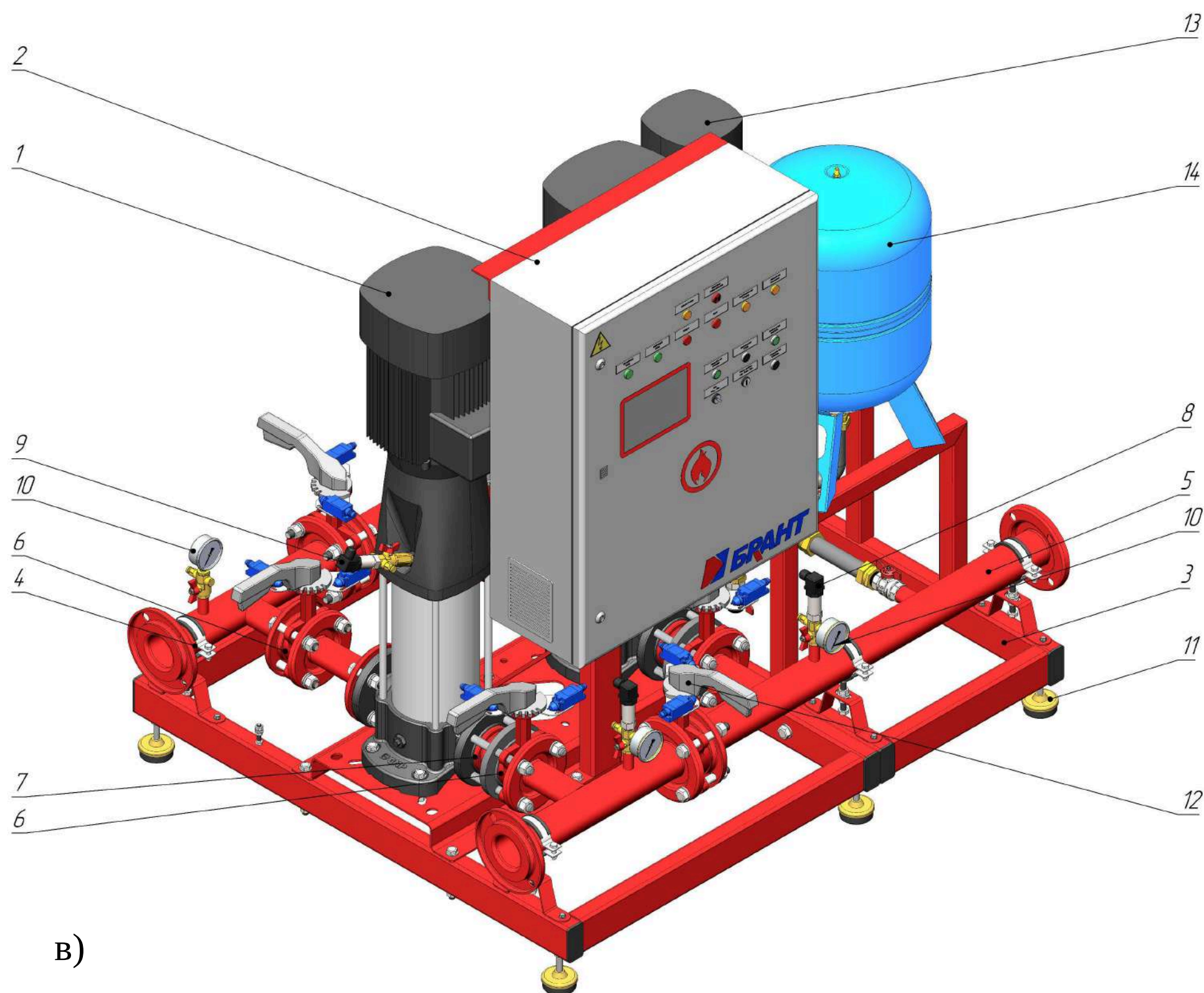
Рисунок – 17. Основное оборудование: а) насосная установка серии АПК:
