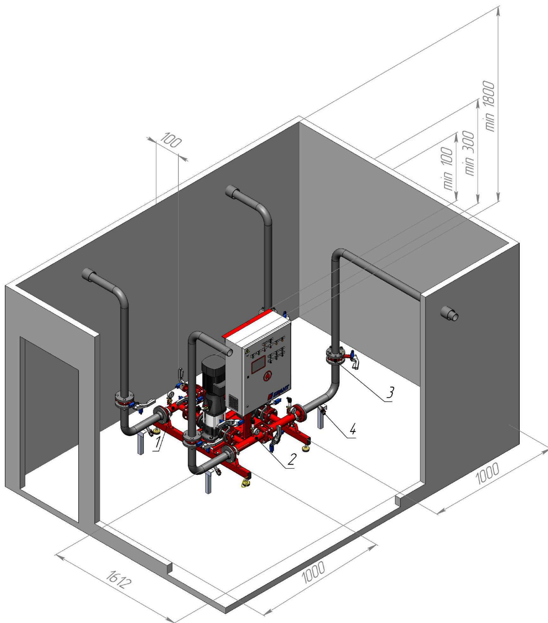
Рисунок – 10. Рекомендуемый вариант подключения насосной установки пожаротушения к водопроводной сети с указанием зон обслуживания и рекомендуемой высоты помещения насосной станции: 1 – коллектор всасывания, 2 – коллектор нагнетания, 3 – запорная арматура, 4 – спускник
